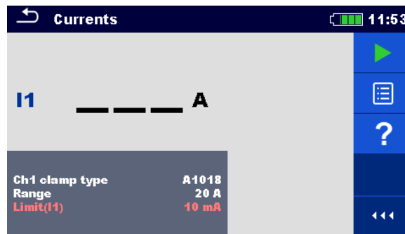
Abbildung 7.59: Menü Strom (I)
