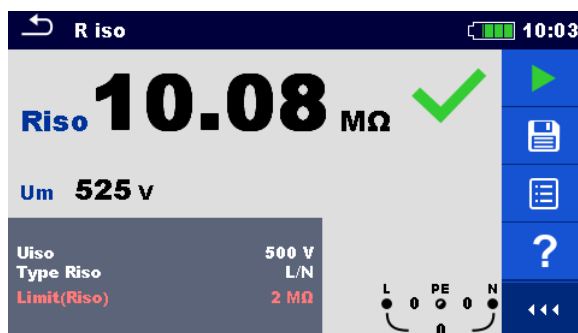
Abbildung 6.1: Bildschirmsicht einer Einzelprüfung, Beispiel für Isolationswiderstandsmessung
