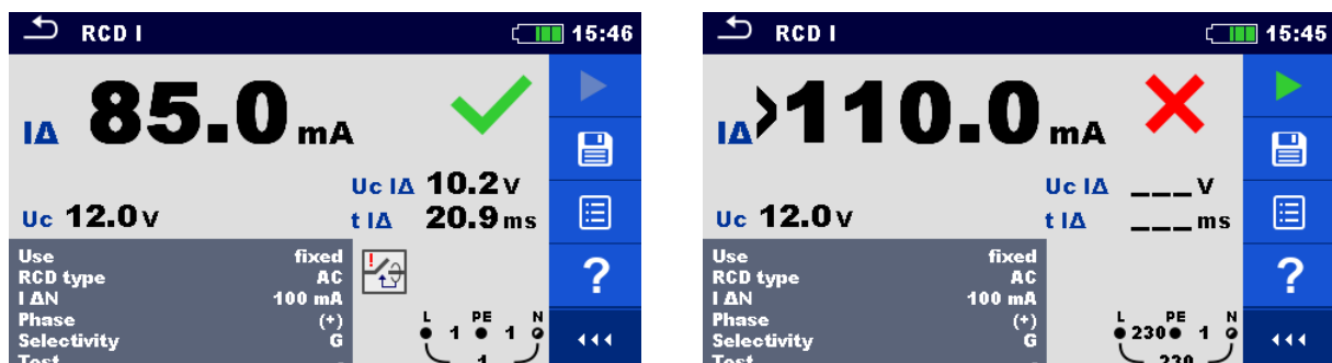
Abbildung 7.28: Beispiele für die Ergebnisse des Auslösestroms
