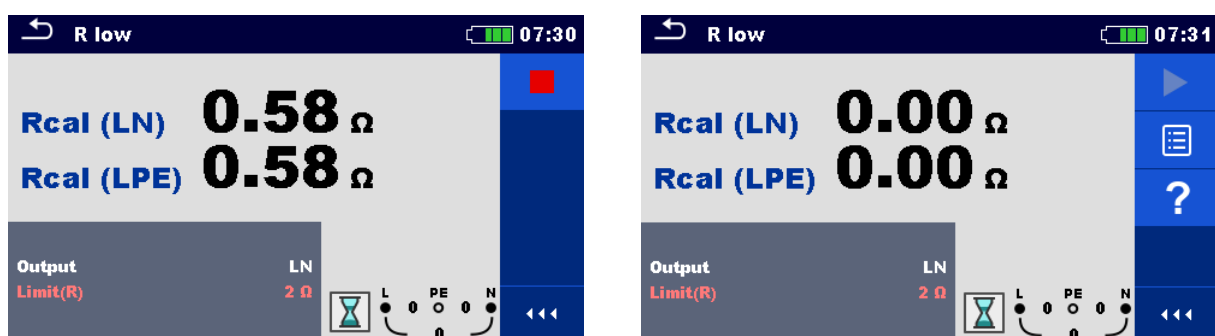
Abbildung 7.23: Ergebnisse vor und nach der Kompensation
