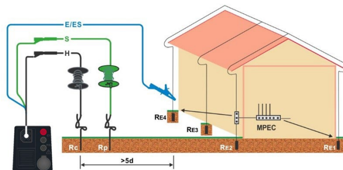
Abbildung 7.48: Erdungswiderstand, Messung einer Blitzschutzanlage mit optionalem Erdungsset (044113)
