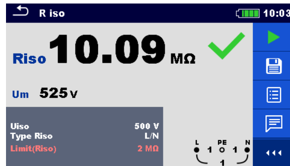
Abbildung 6.4: Ergebnisbildschirm einer Einzelmessung, Beispiel für Isolationswiderstandsmessung
