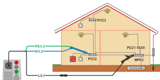
Abbildung 7.17 Anschluss der 3-Leiter-Prütleitung und der optionalen 40 m Messleitung BENNING TA 5 (044039)
