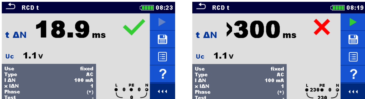
Abbildung 7.27: Beispiele für die Ergebnisse der Auslösezeit
