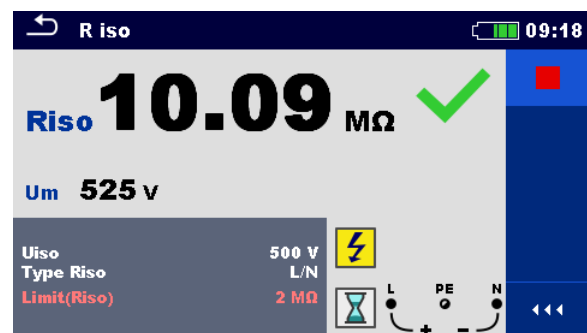
Abbildung 6.1: Bildschirmsicht einer Einzelprüfung, Beispiel für Isolationswiderstandsmessung
