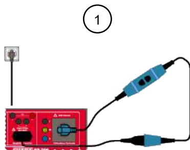
Abb. 28: PRCD prüfen (Anschlussschema)
