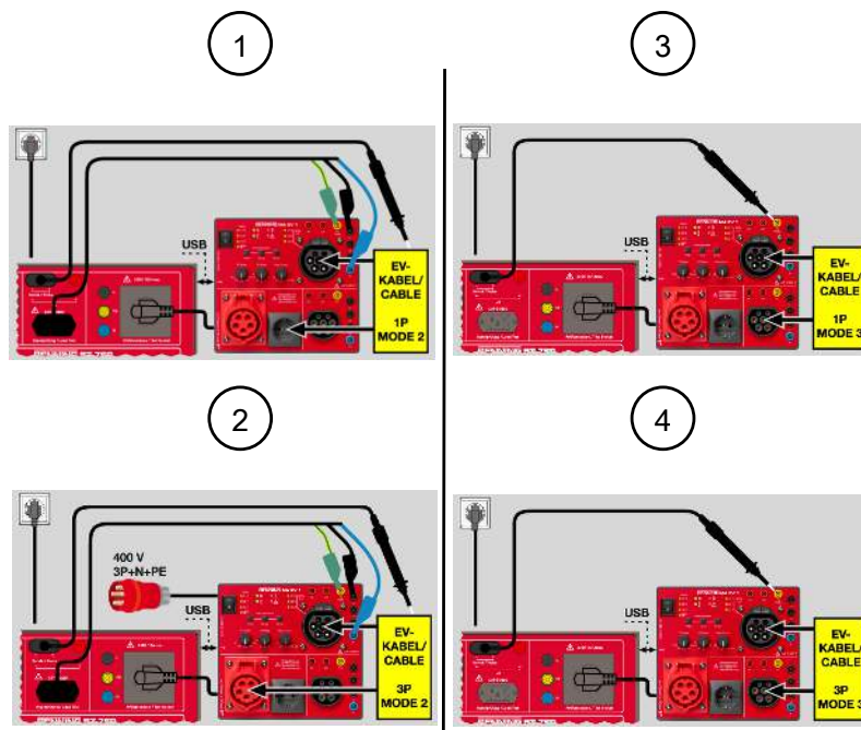
Abb. 29: EVSE prüfen (Anschlussschema Prüfaufbau EVSE Prüfungen)
