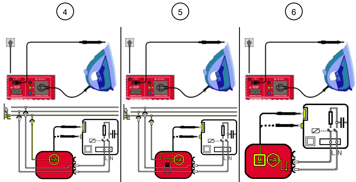
Abb. 19: Berührungstrom prüfen SK II (Anschlussschema beispielhaft für VDE 0701 und VDE 0702, Stromlaufplan)
