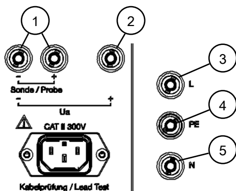
Abb. 12: Geräteansicht-Buchsen
