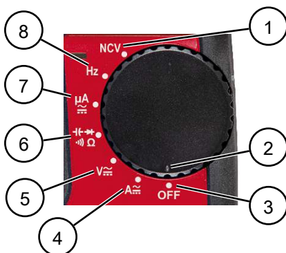
Afbeelding 2: Draaischakelaar
