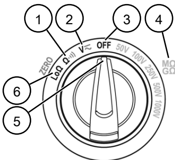
Afbeelding 2: Draaischakelaar
