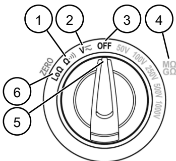
Illustration 2: Commutateur rotatif
