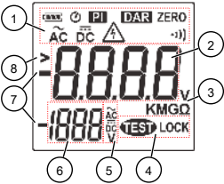
Afbeelding 3: Digitaal display
